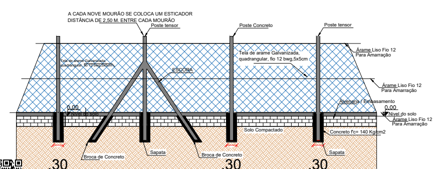
VISTA FRONTAL ALAMBRADO
