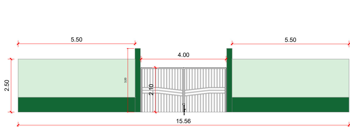
FACHADA ESC. 1/ 55
