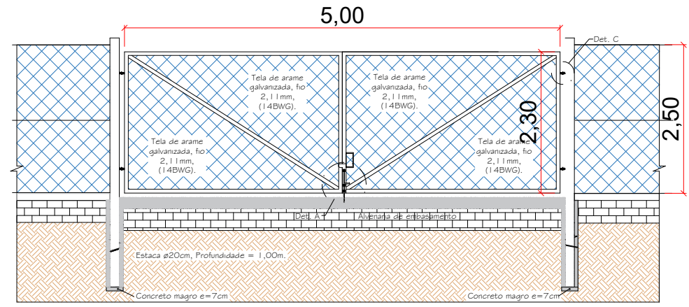
DETALHE PORTÃO 1
