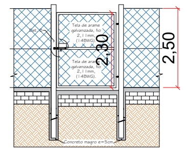
DETALHE PORTÃO 2
